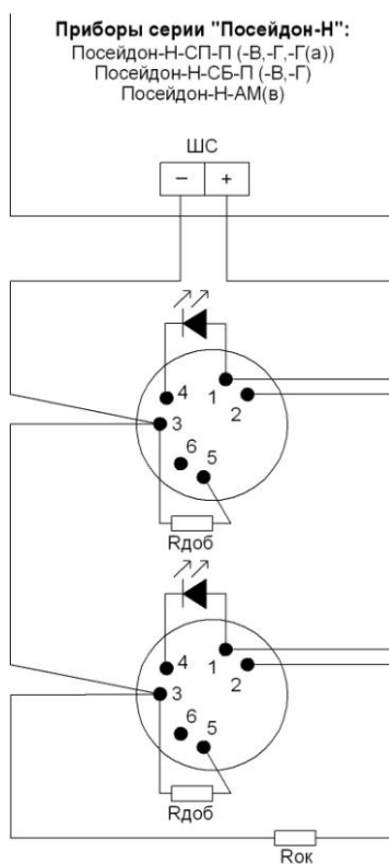
Подключение YBN-R/6M к приборам серии «Посейдон-Н» (неэкранированный кабель)
