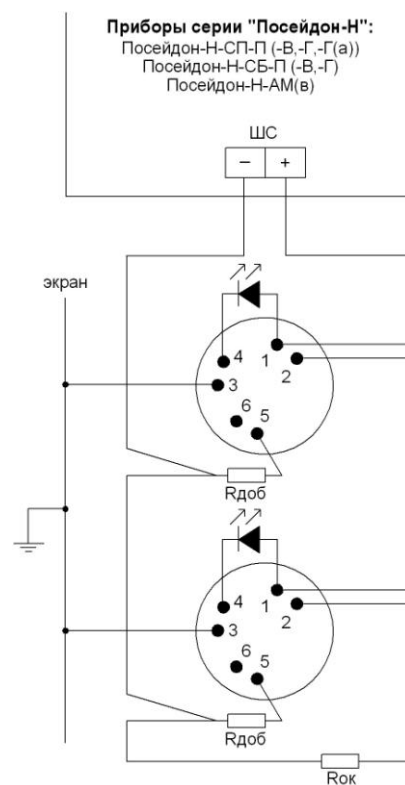
Подключение YBN-R/6M к приборам серии «Посейдон-Н» (экранированный кабель)
