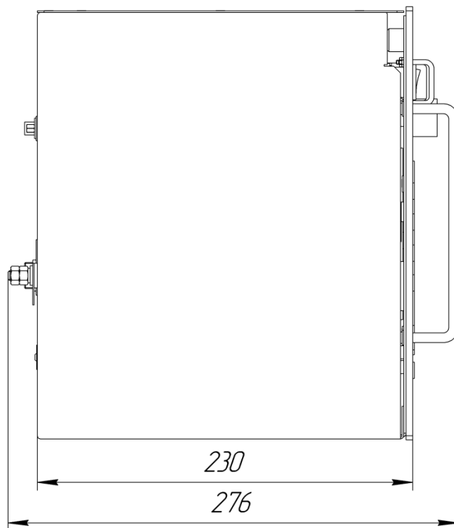
Рисунок 2 - Внешний вид прибора, в стойку 19”
