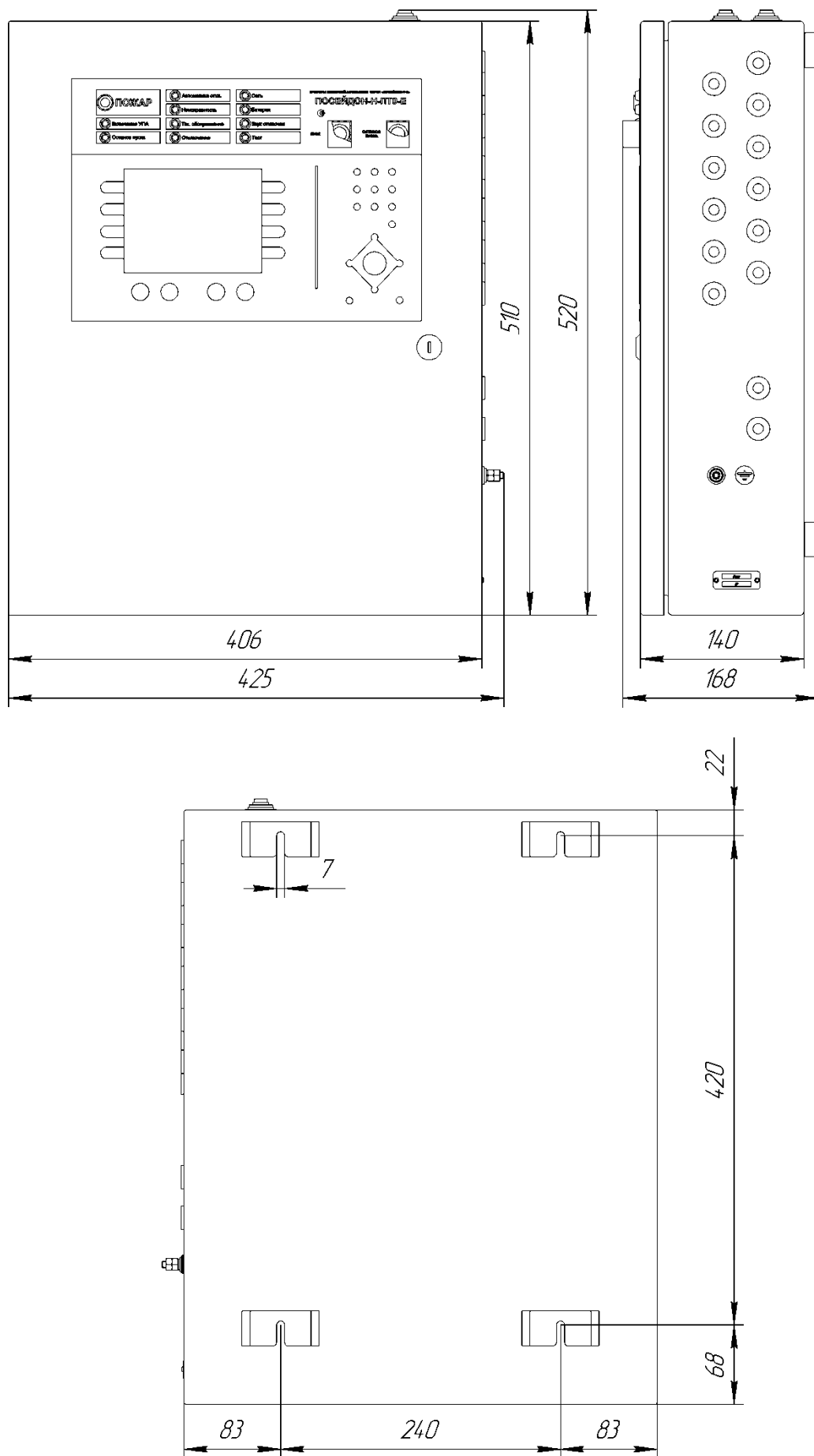
Рисунок 1 - Внешний вид прибора, в настенном исполнении
