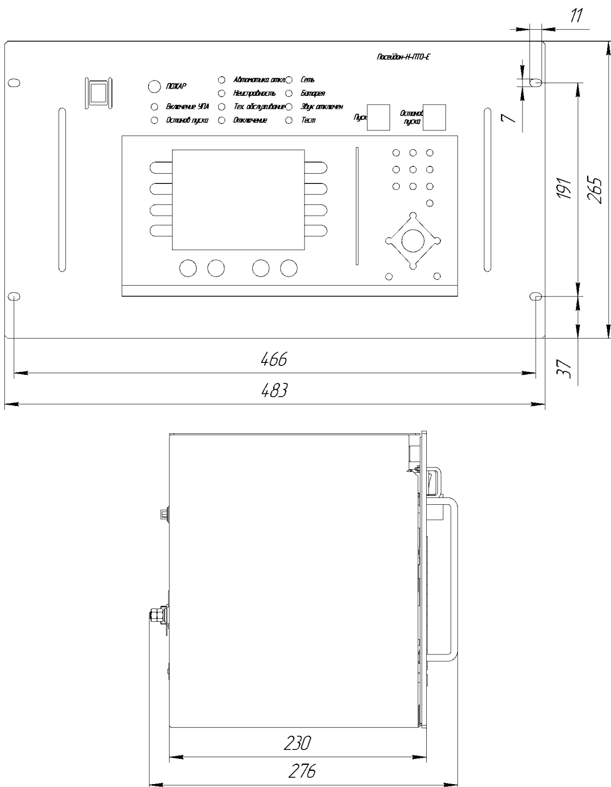
Рисунок 2 - Внешний вид прибора, при исполнении в стойку 19”
